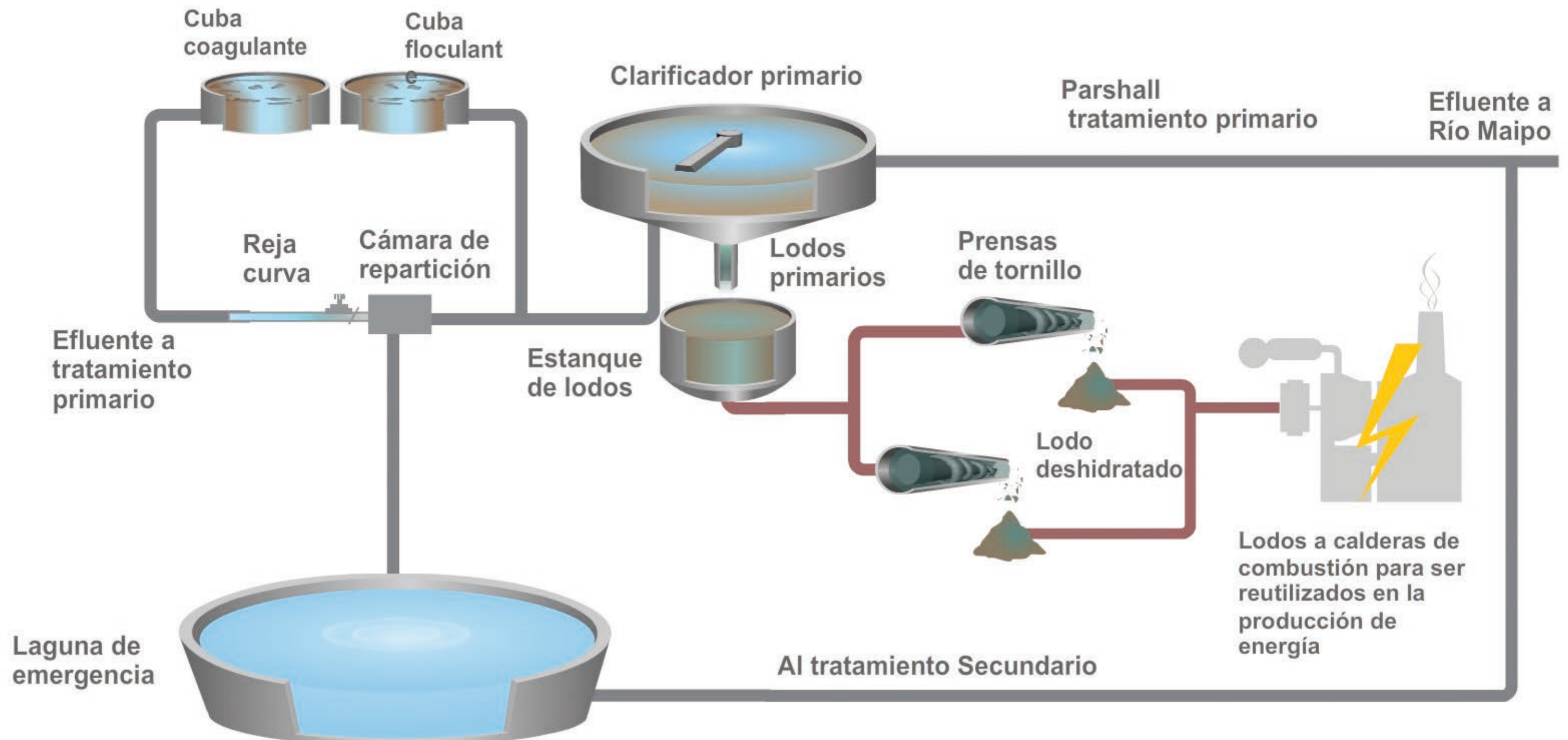
Diagrama Sistema de tratamiento primario.
