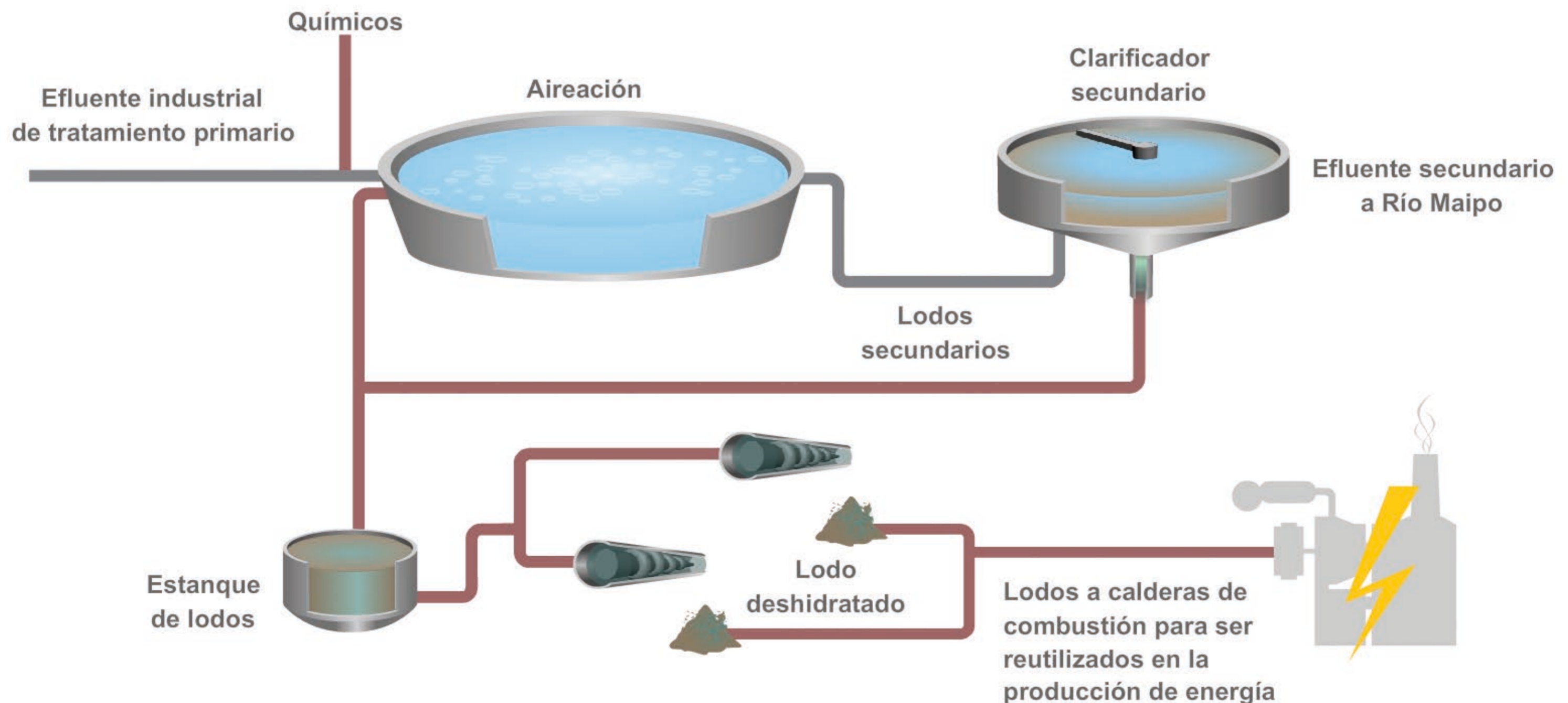
Tratamiento secundario de Riles.
